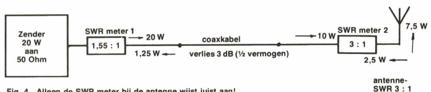
Fig. 4 Alleen de SWR meter bij de antenne wijst juist aan!
