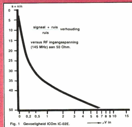
Fig. 1 Gevoeligheid ICOM IC-02E
